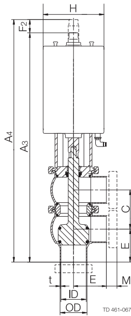
Válvula de desvio
