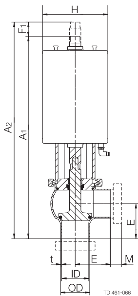
Válvula de fechamento
