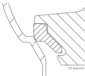
Vedação do assento PTFE (TR2)
